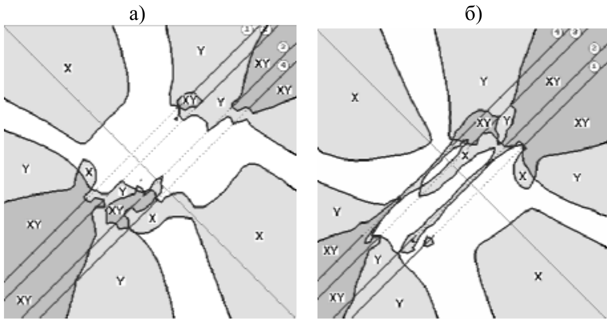
Рис. 3. Границы зон опорного давления при отработке свиты пластов: а) при нисходящем порядке отработки; б) при восходящем порядке отработки
