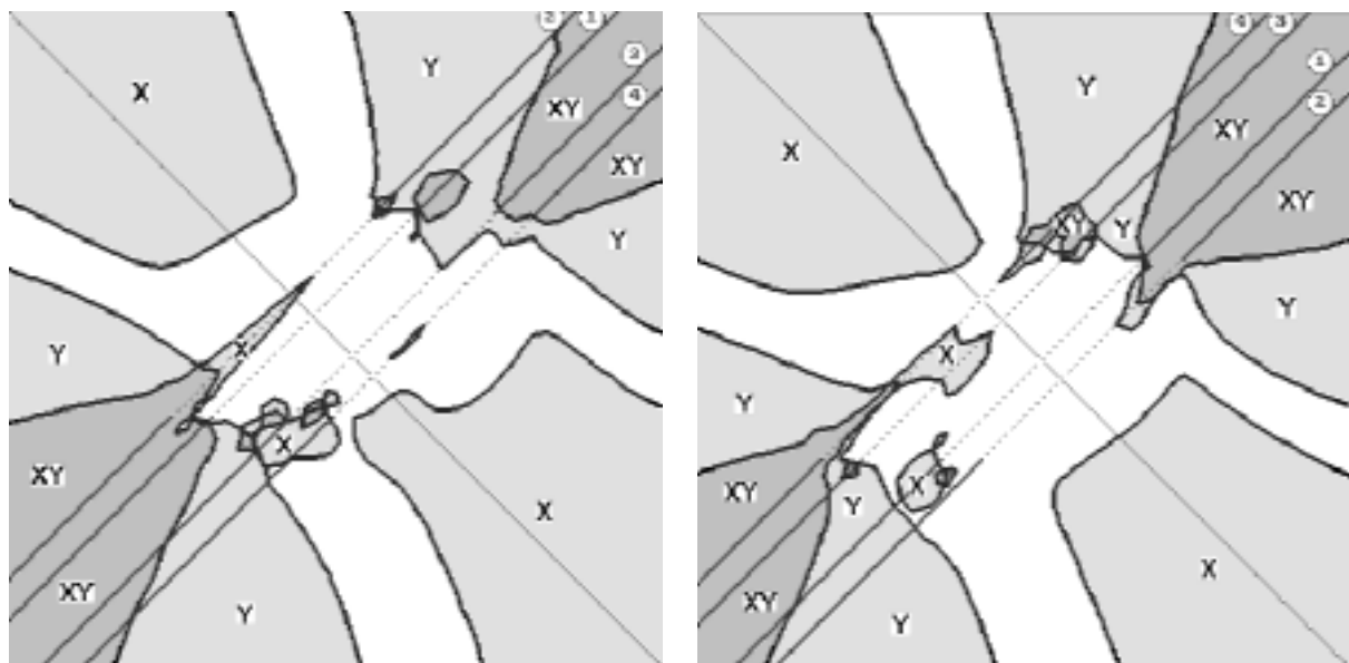
Рис. 4. Границы зон опорного давления при комбинированном порядке отработки свиты пластов: а) с первичной надработкой нижележащих пластов; б) с первичной подработкой вышележащих пластов
