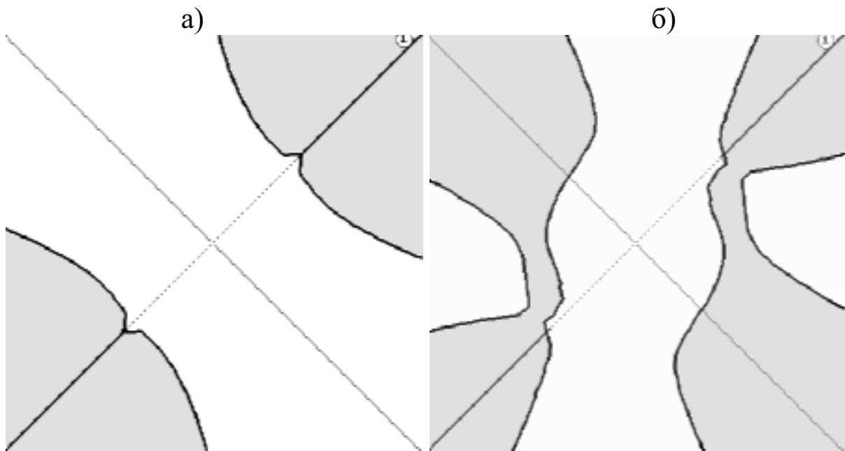
Рис. 1. Границы зон опорного давления для одиночной лавы, построенные: а) по критерию \sigma_{yy} = 0 ; б) по критерию \sigma_{xx} = 0
