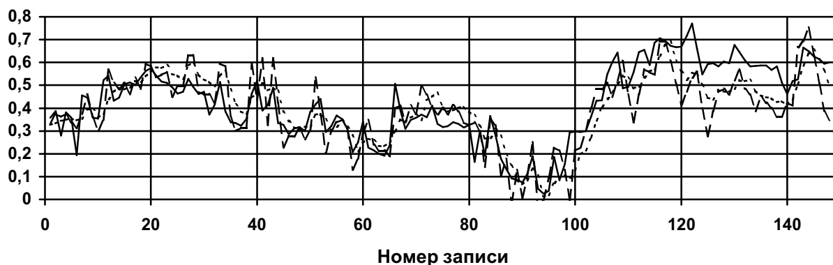
Рис. 1. Нормированное фактическое и прогнозируемое суточное потребление газа. а) тренировочные данные за 1996—1997 гг.; б) контрольная выборка за 1998 г.; кривая «—» — G^* ; кривая «— — —» — \hat{G}^* ; кривая «- - -» — \hat{G}_h^*
