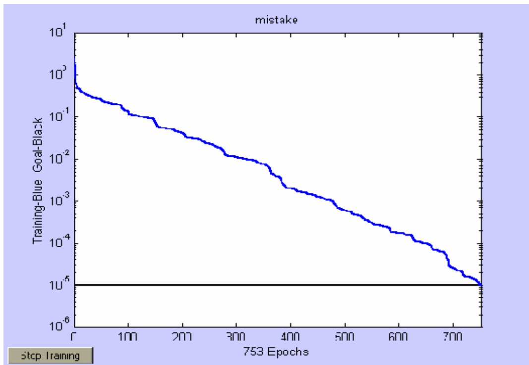
Рисунок 3.- Процес навчання.
