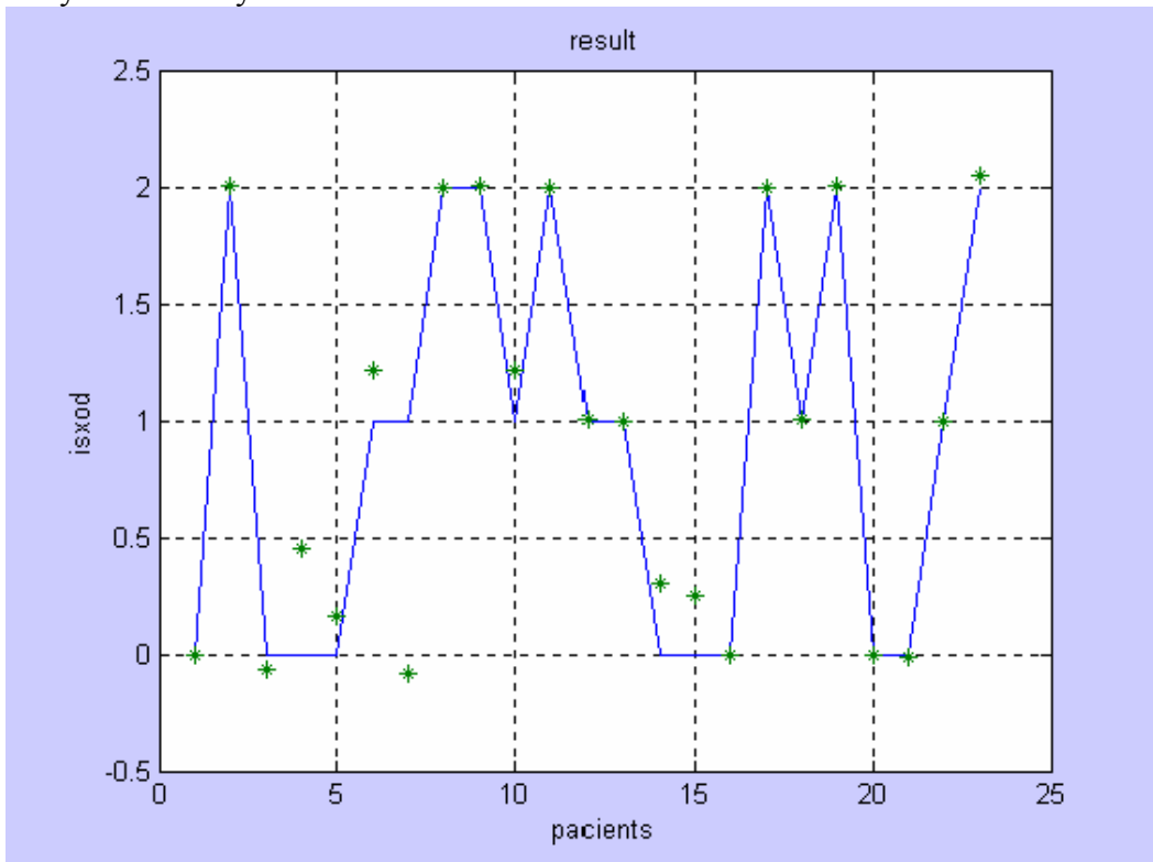
Рисунок 5.- Тестування мережі.
