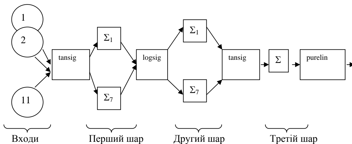
Рисунок 2. Архітектура мережі.
