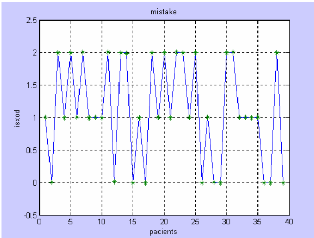
Рисунок 4.- Результат навчання.
