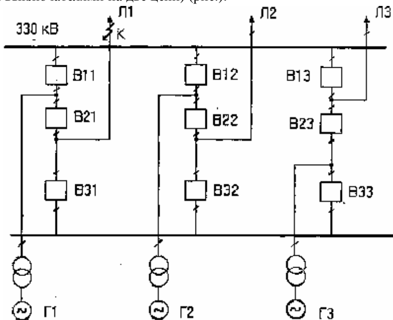
Рисунок - Полуторная схема соединений
