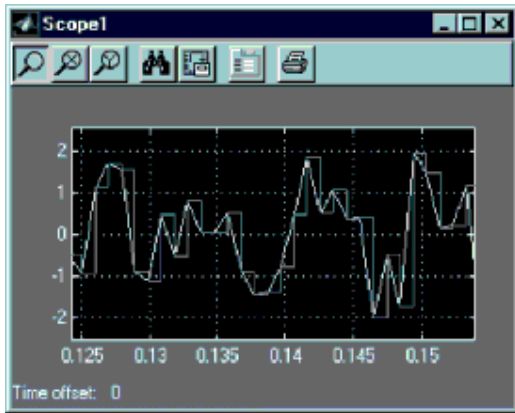
Рис. 10. Фрагменты входного и выходного сигналов АЦП
