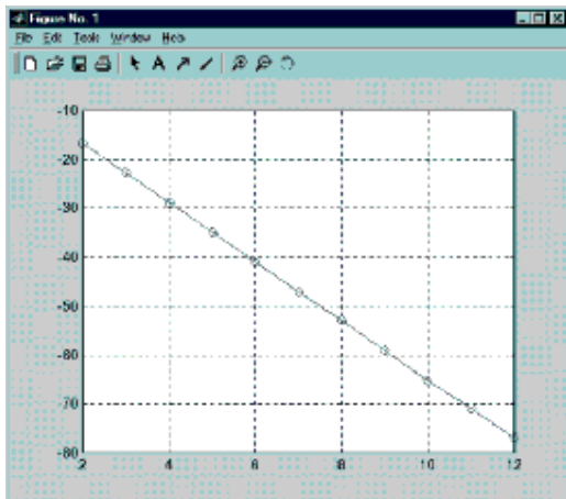
Рис. 11. Зависимость дисперсии шума квантования от разрядности АЦП
