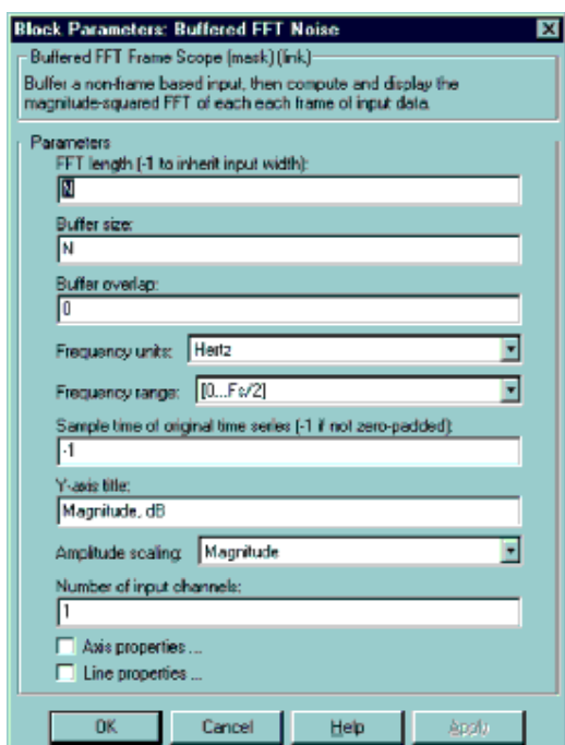
Рис. 6. Окно и значения параметров блока Buffered FFT Frame Scope
