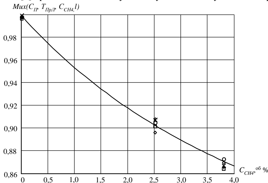
Рисунок 5 – Залежність Mux(C_{\text{П}}, T_{\text{Прл}}, C_{\text{СН}_4}, l) від зміни концентрації метану у діапазоні від 0 до 4 об.% при зміні C_{\text{П}} та T_{\text{Прл}}
