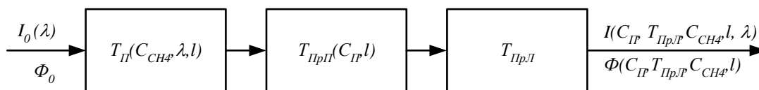
Рисунок 1 – Фактори, які призводять до зміни оптичної потужності випромінювання у відкритому оптичному каналі вимірювача
