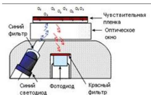
Р и с. 1. Конструкция головки измерителя, основанного на динамической Люминесценции
