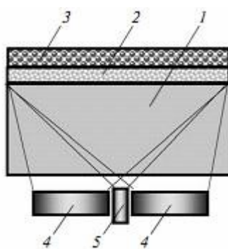
1 — кварцевое стекло; 2 — люминесцентное покрытие; 3 — светозащитная мембрана; 4 — измерительный и опорные фотодиоды; 5 — светодиод [5]
