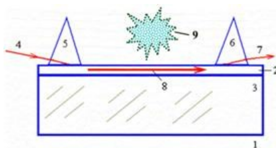
1 – воздух; 2 – волноводный слой (пленка); 3 – подложка; 4, 7 – вводимое и выводимое излучение; 5, 6 – призмы; 8 – направленная волноводная мода; 9 – исследуемая среда [7]
