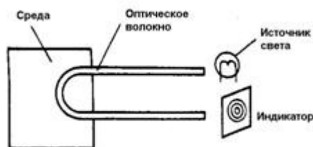
Р и с. 6. Структура двухмодового волоконно-оптического датчика
