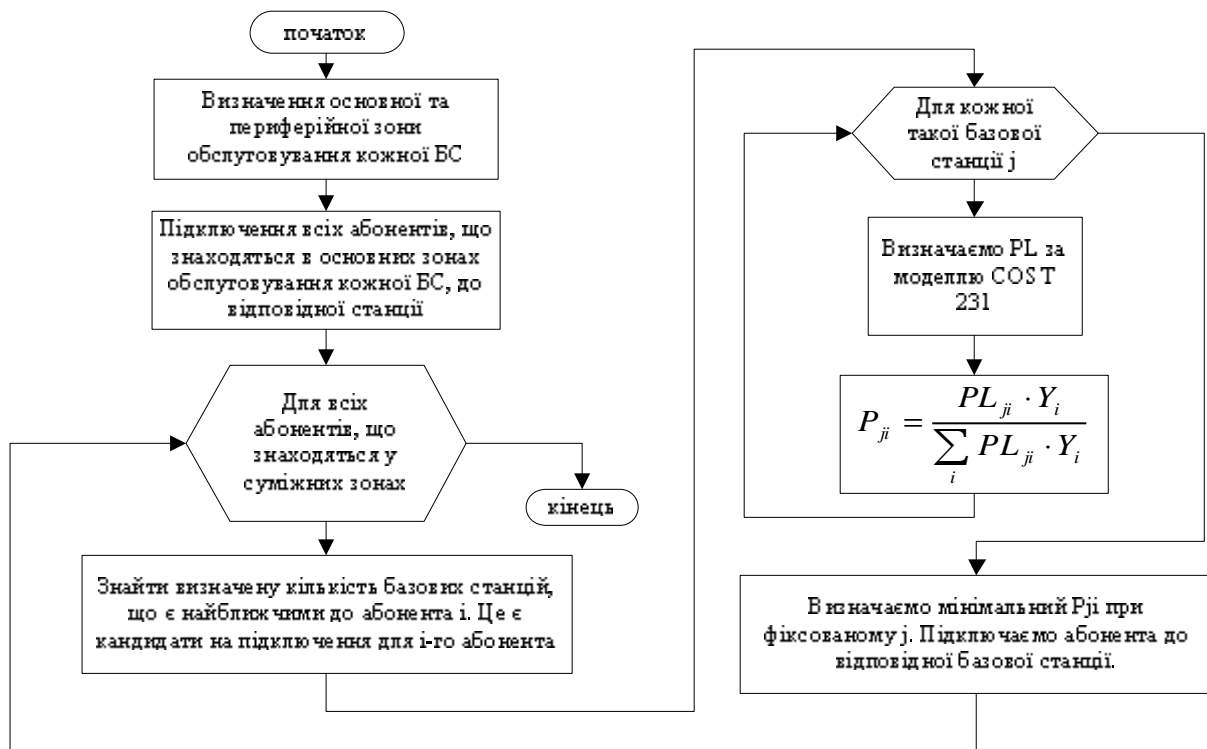
Рисунок 2 - Алгоритм перерозподілу абонентів по БС
