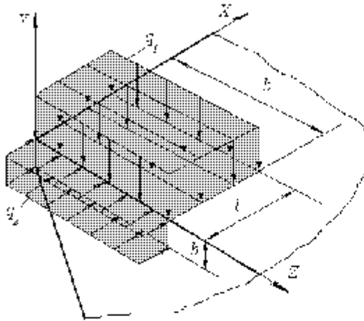
Рис. 1. Схема действия тепловых потоков на передней и задней поверхностях лезвия режущего инструмента
