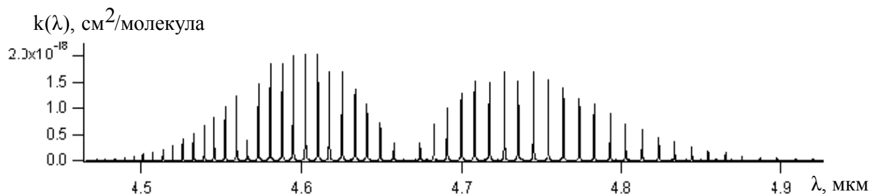
Рисунок 2 – Наиболее интенсивная полоса спектра поглощения угарного газа
