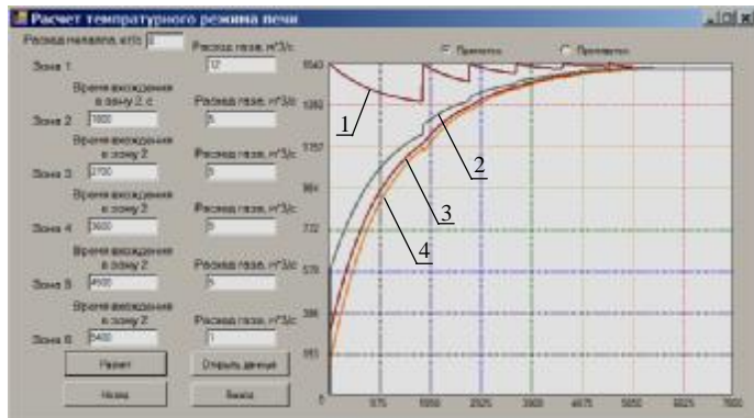
Рисунок 2 – Окно расчета температурного режима печи
