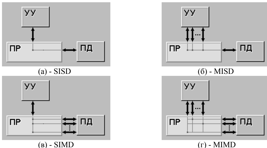
Рис. 1. Виды архитектур по Флинну
