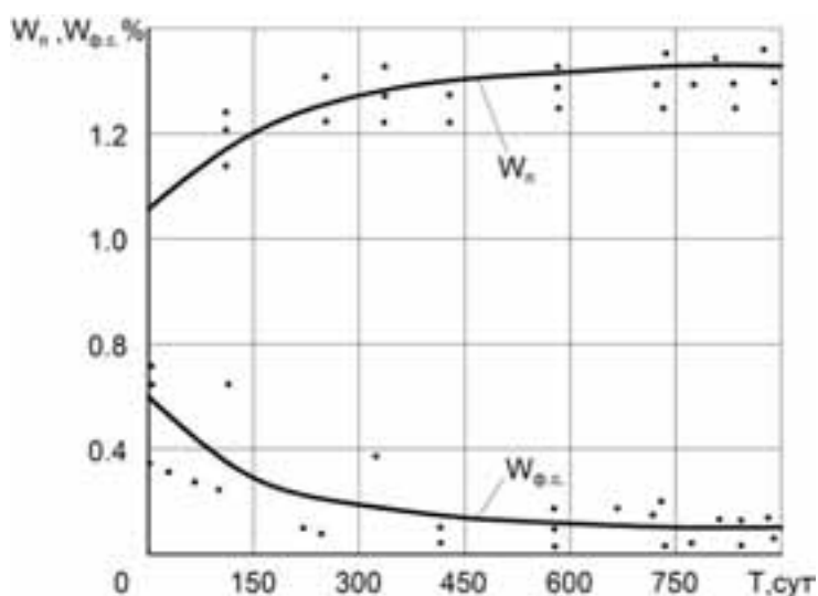
Рис.1 Зависимости полной влагоемкости W_n и физически связанной влажности W_{ф.с.} от времени T образцов осадочных горных пород
