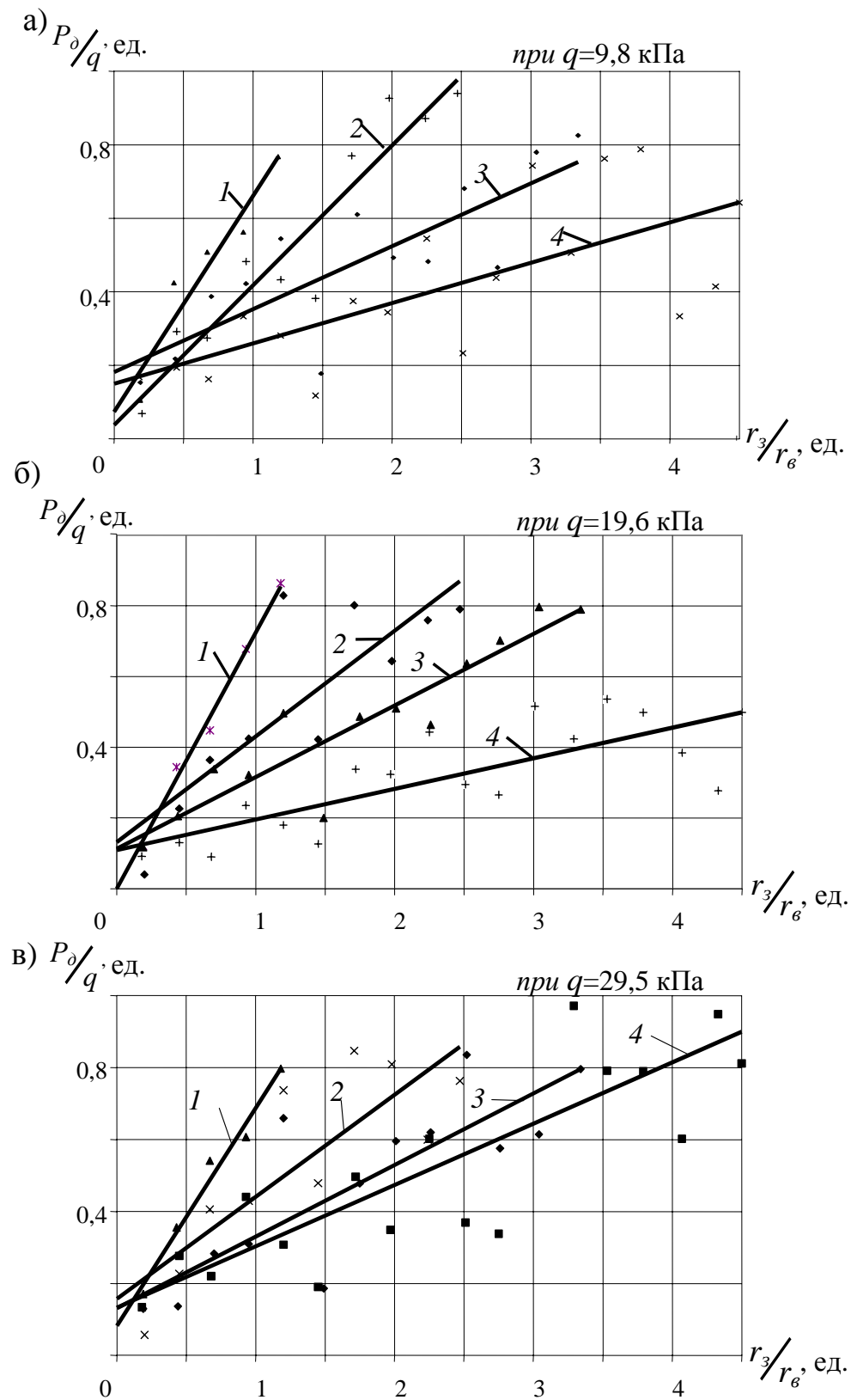
Рис. 3. Графики изменения вертикального давления P_d в пределах ЗРП на уровне почвы выработки при различных значениях внешней пригрузки q и радиуса зоны r_3 (1, 2, 3, 4 – соответственно при радиусе ЗРП: 1,2; 2,5; 3,4; 4,6 r_8 )
