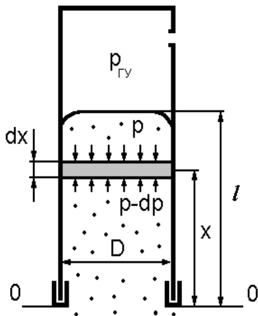
Рис.2. Схема к расчету глубины разрушения монолита
