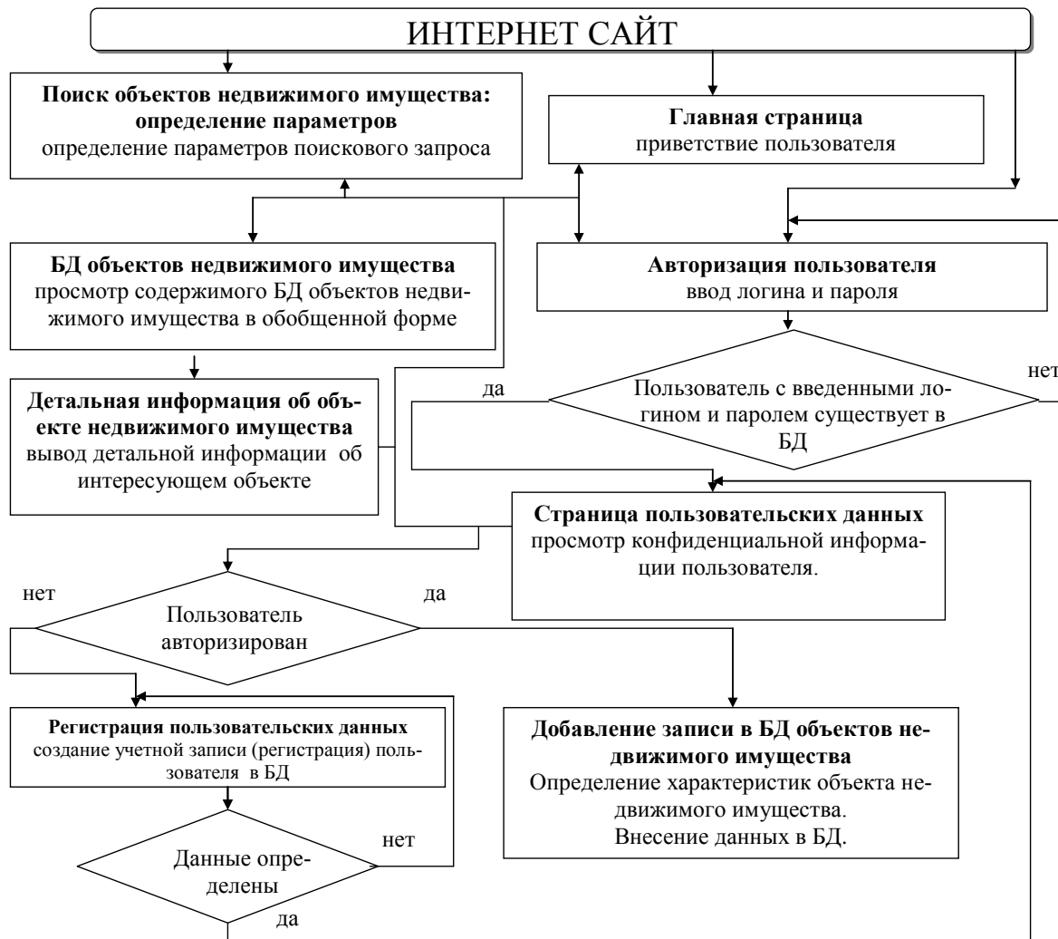
Рисунок 3 - Логическая структура Интернет ресурса
