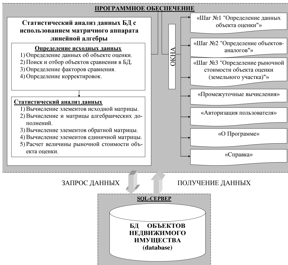
Рисунок 4 - Модель программного обеспечения
