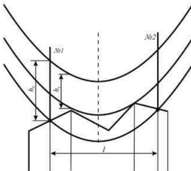
Рис. 2. Ілюстрація дотику габаритної кривої точки зламу повздовжнього профілю
