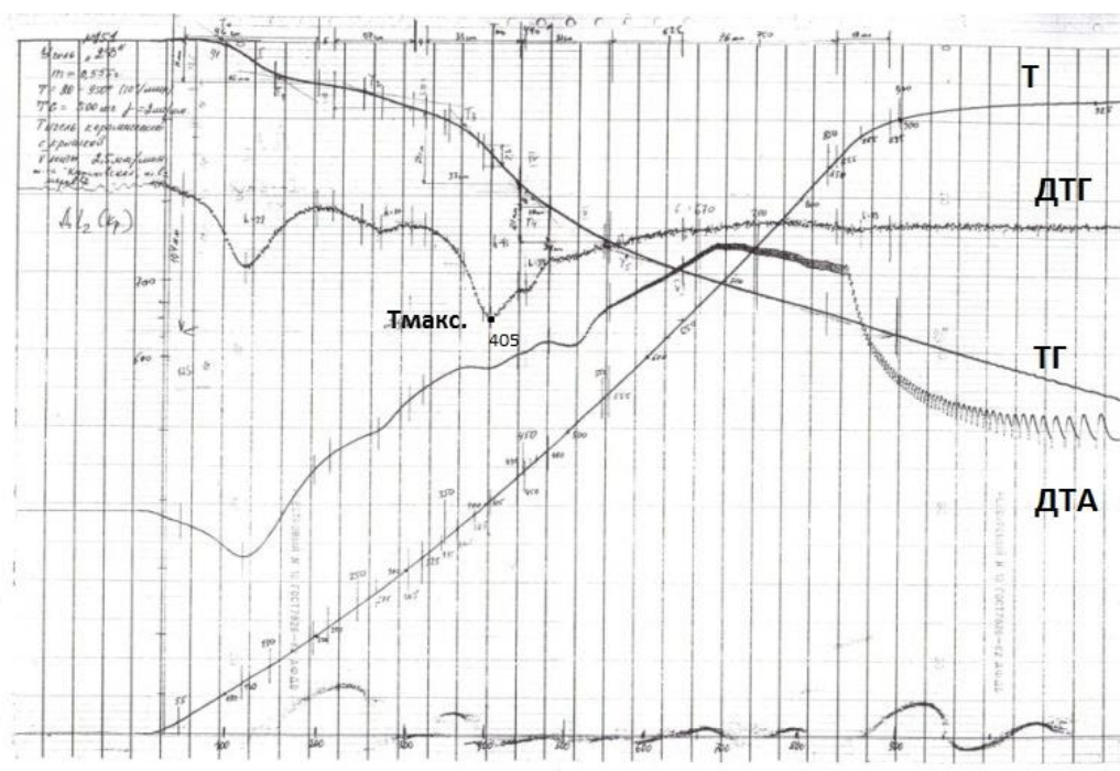
Рис. 1 – Дериватограмма исследуемого угля
