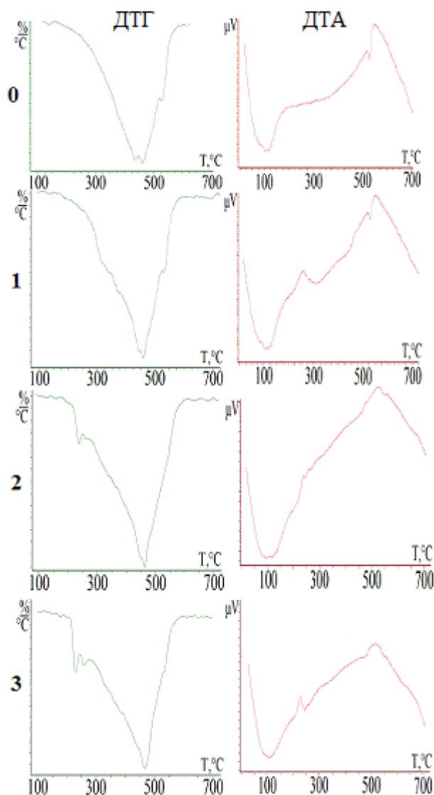
Рисунок 3 – Термічний аналіз пеків, модифікованих ПВХ. Кількість ПВХ: 1– 1%; 2– 3%; 3– 5% (швидкість нагрівання 10°C/хв).
