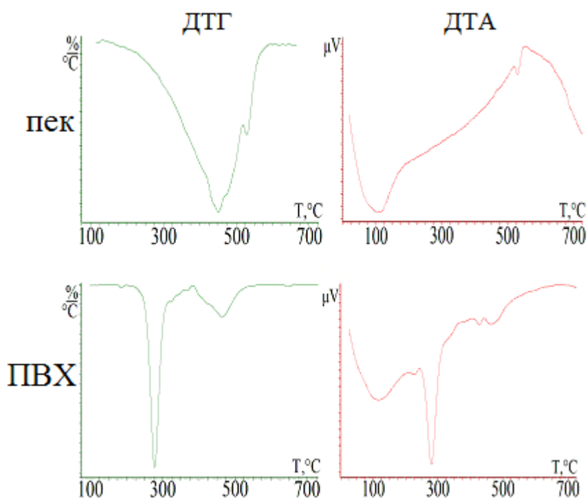
Рисунок 1 – Термічний аналіз вихідного кам'яновугільного пеку та ПВХ (швидкість нагрівання 10°C/хв).
