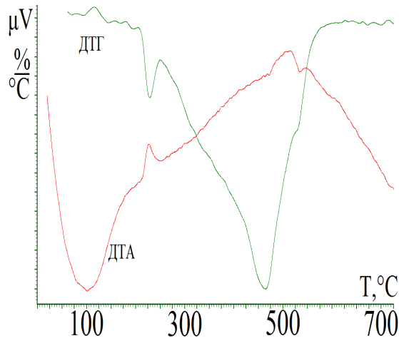
Рисунок 2 – Термічний аналіз суміші компонентів вихідний пек – ПВХ (3%) (швидкість нагрівання 10°C/хв).
