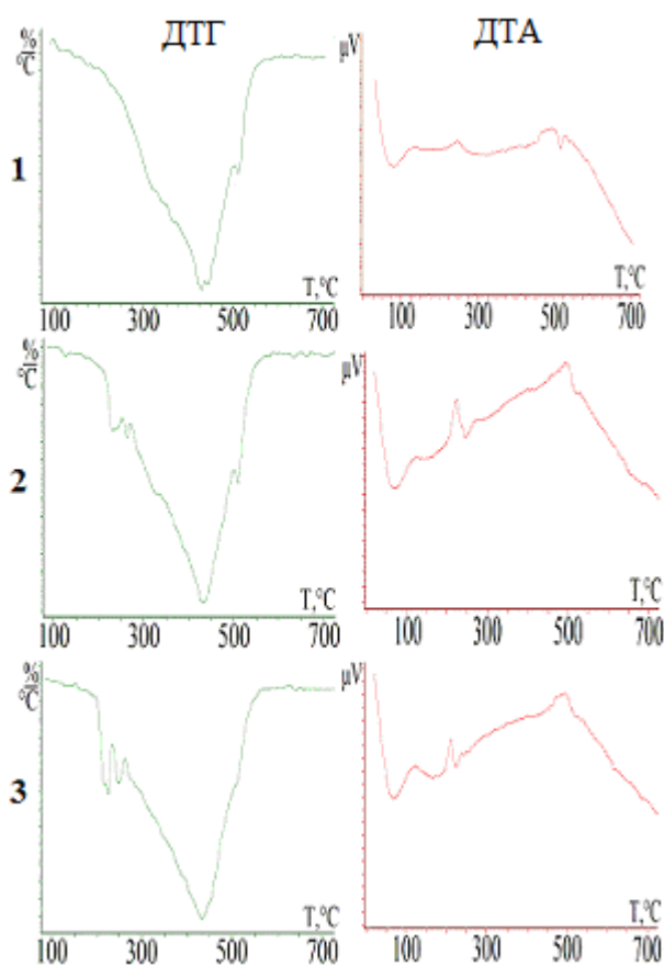
Рисунок 4 – Термічний аналіз пеків, модифікованих ПВХ. Кількість ПВХ: 1– 1%; 2– 3%; 3– 5% (швидкість нагрівання 5°C/хв).
