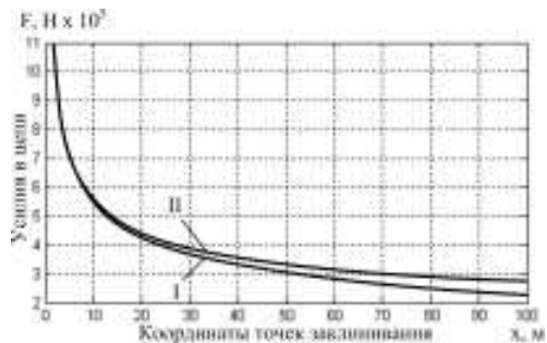
Рисунок 4 – Зависимость максимальной величины динамических усилий в цепи от места заклинивания: I – одноприводной; II – двухприводной
