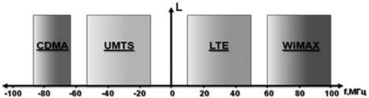
Рисунок 4 - Сигнали після перенесення в область роботи АЦП
