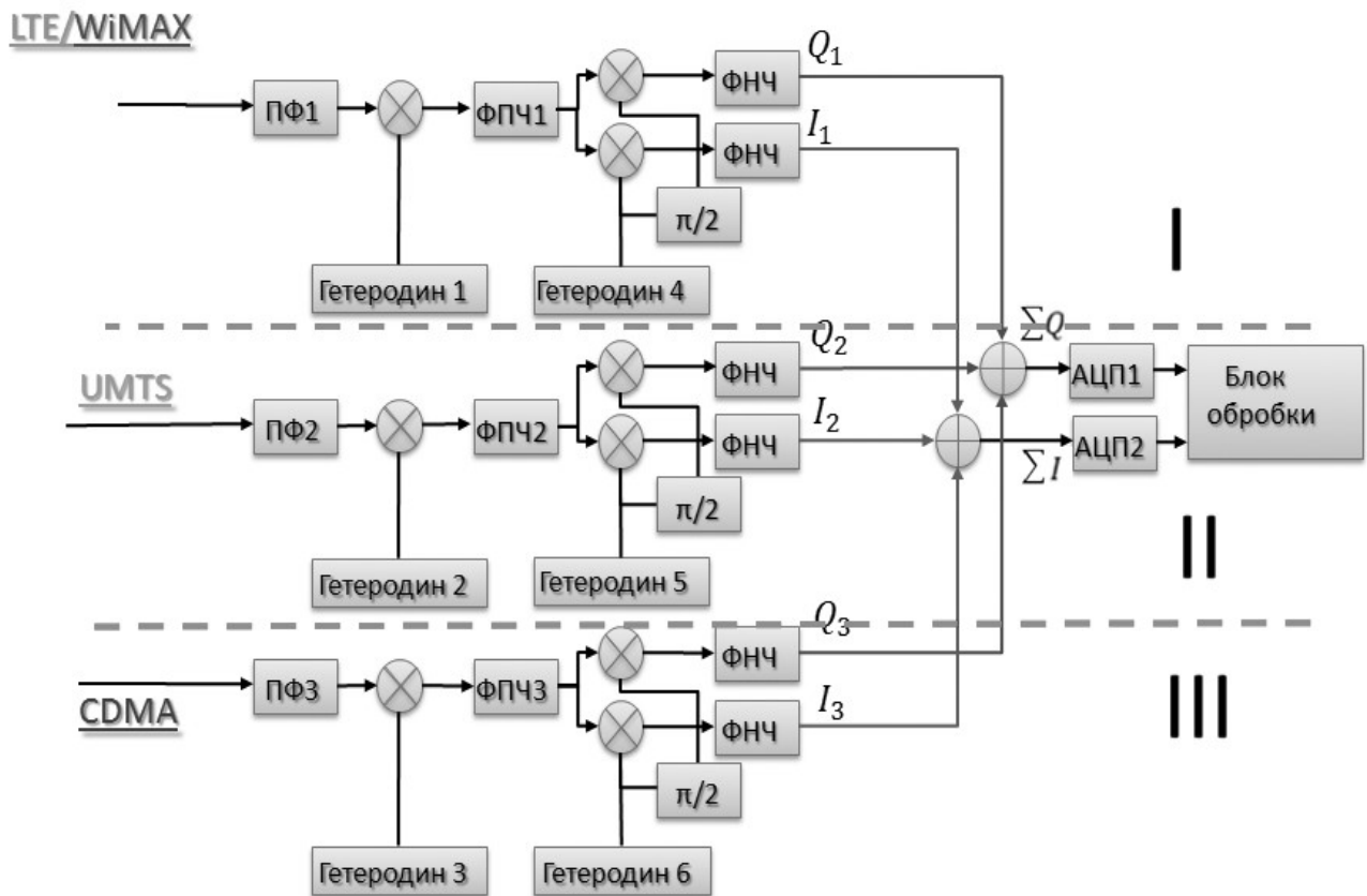
Рисунок 1 – Структурна схема multi-MSP 1-го рівня
