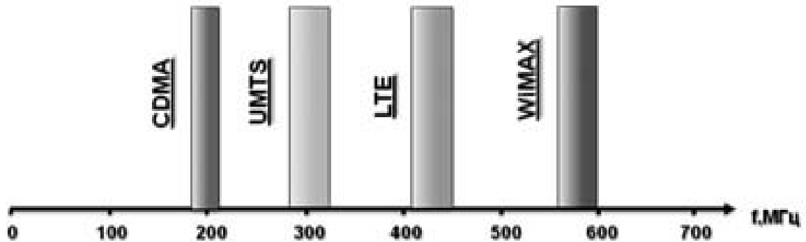
Рисунок 3 - Розташування всіх сигналів в частотному діапазоні після першого переносу в мегагерцовий діапазон
