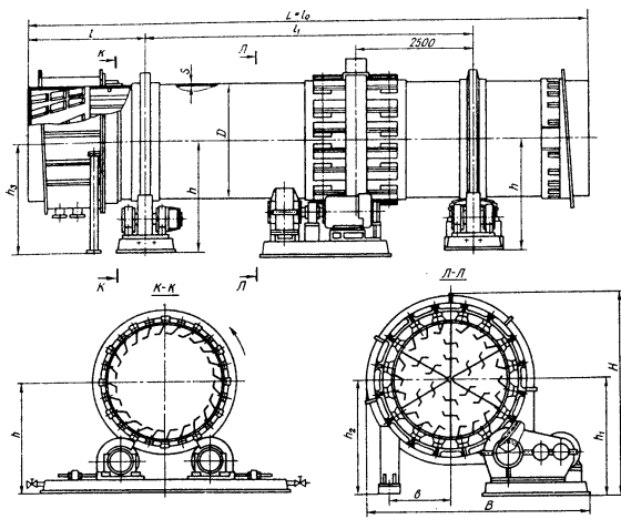
Рис. 47.7. Барабанная вращающаяся сушилка типа БН диаметром 2500—3500 мм
