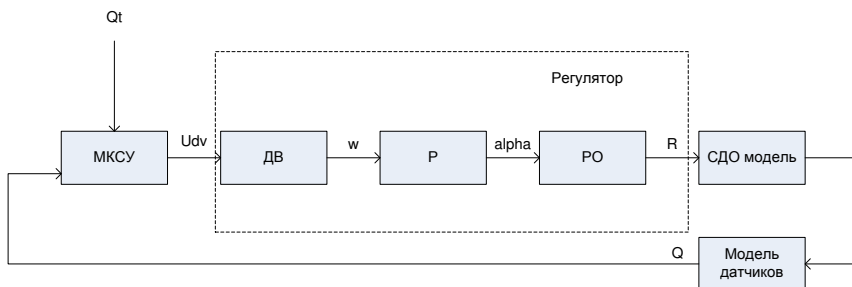
Рисунок 3 - Структура регулятора
