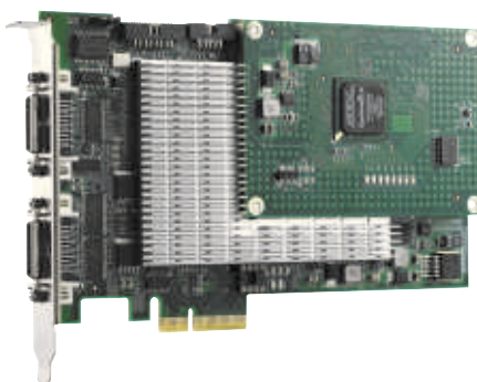
Рис. 4. Плата PCIe-CML64F с интерфейсом Camera Link®
