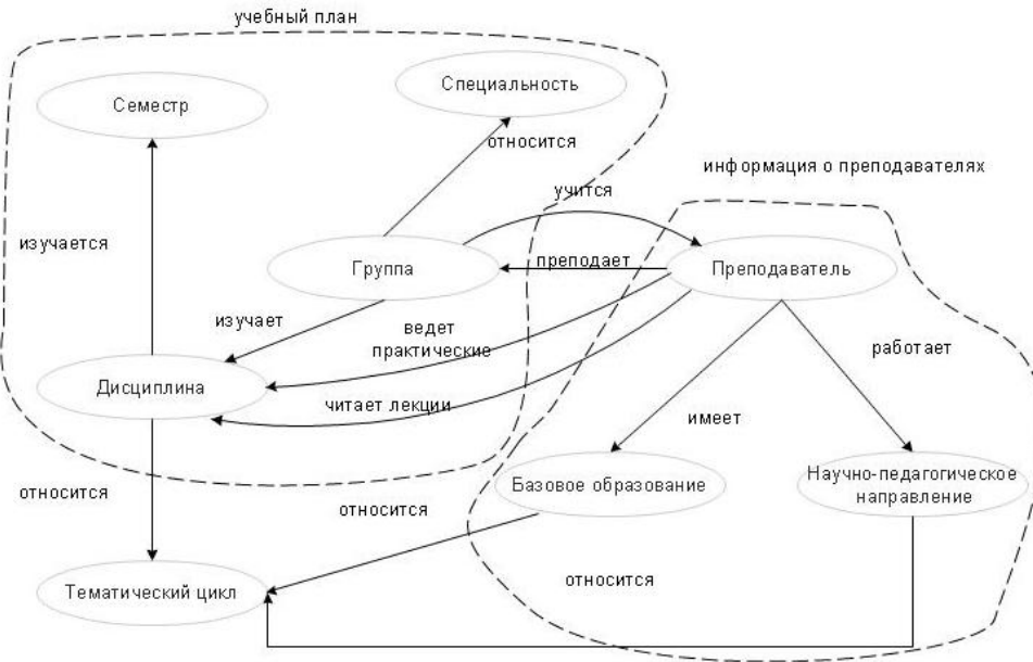
Рис. 1. Семантическая модель данных
