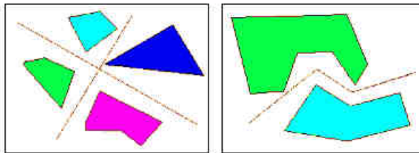
Рис. 1. Линейно и нелинейно делимые классы
