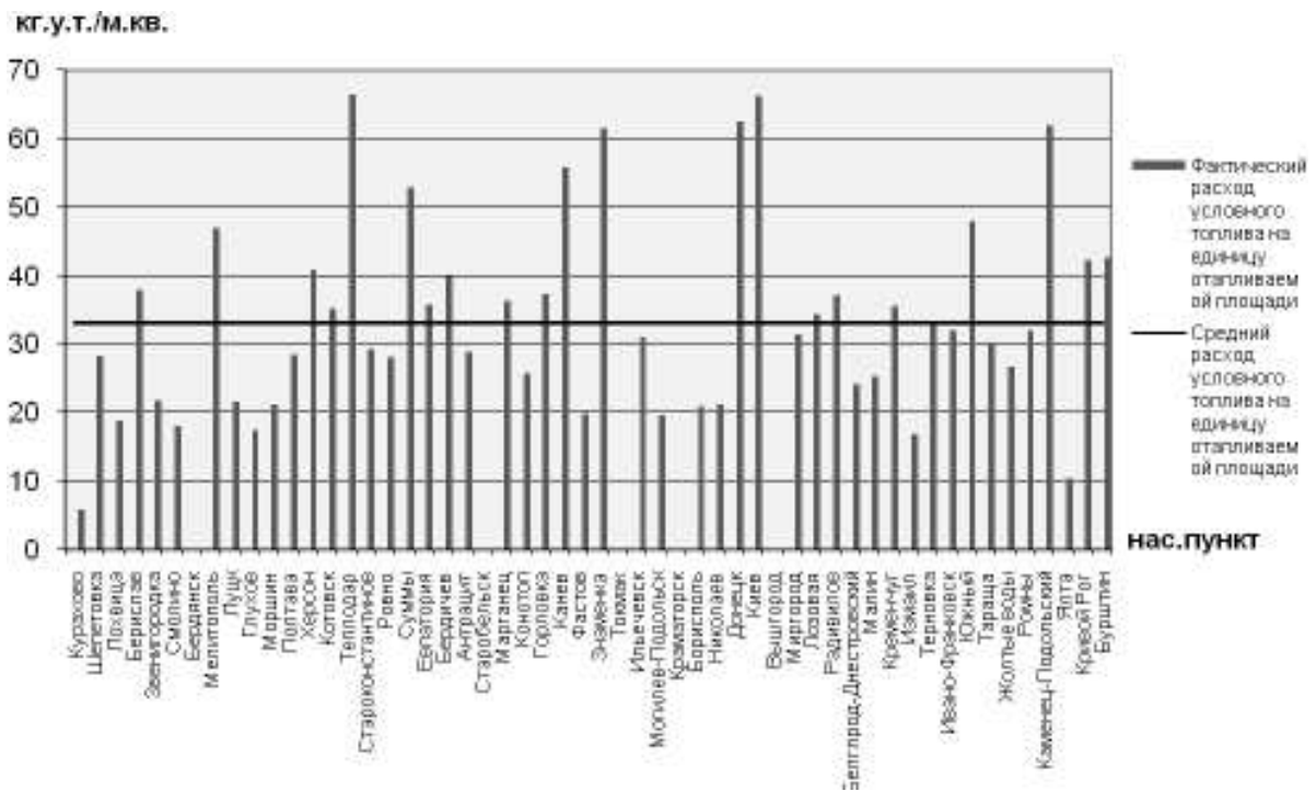
Рис. 8. Фактический удельный (на единицу отапливаемой площади) расход условного топлива по городам Украины
