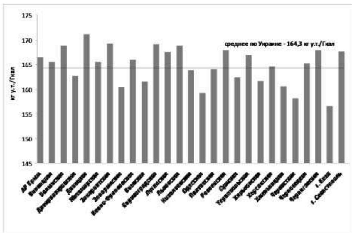
Рис. 5. Удельные затраты топливно-энергетических ресурсов на выработку тепловой энергии по областям Украины в первом полугодии 2010 года
