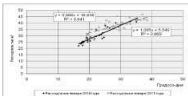
Рис. 11. Зависимость расхода природного газа котельной от градусо-дней за январь 2010 г. и январь 2011 г.
