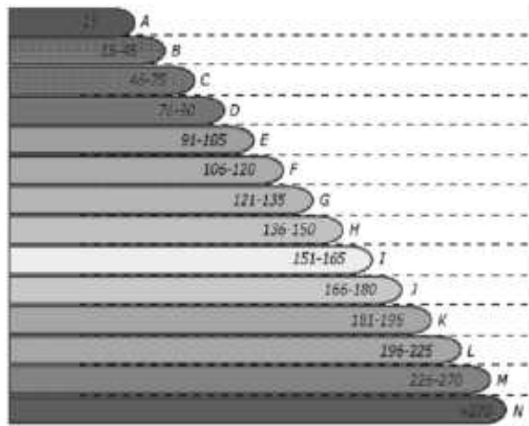
Рис. 7. Стандартизированное потребление тепловой энергии, кВт·ч/м 2 за год
