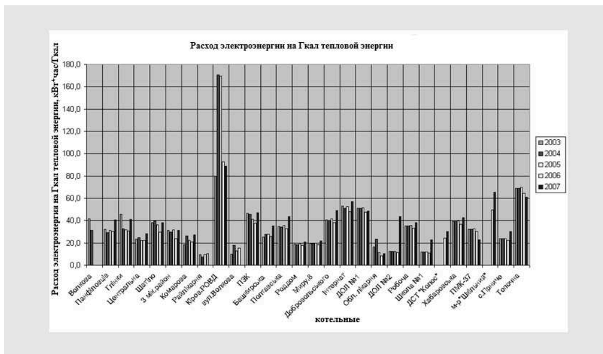
Рис. 9. Удельные затраты электроэнергии на транспортировку теплоносителя
