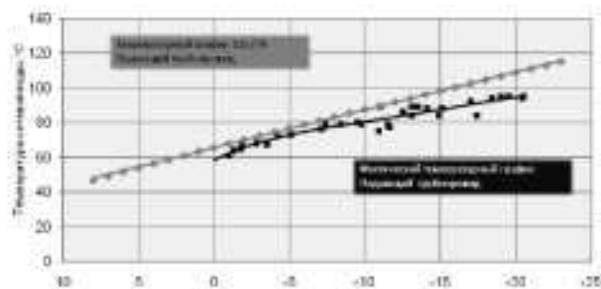
Рис. 10. Сравнительный график температур теплоносителя в подающем трубопроводе
