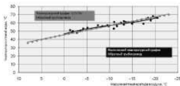
Рис. 10а. Сравнительный график температур теплоносителя в обратном трубопроводе
