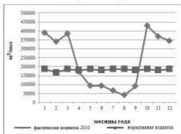
Рис. 15. Динамика нормативного и фактического использования подпиточной воды за год
