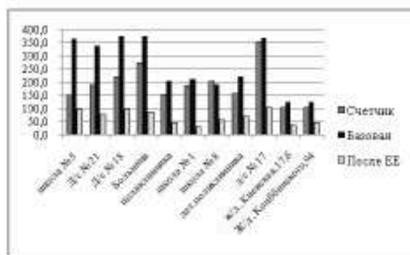
Рис. 6. Удельное энергопотребление зданий (кВт·ч/(м²·год))
