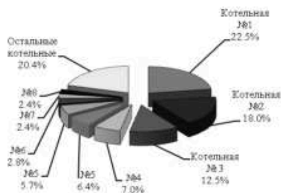
Рис. 2. Распределение присоединенной тепловой нагрузки между тепловыми источниками
