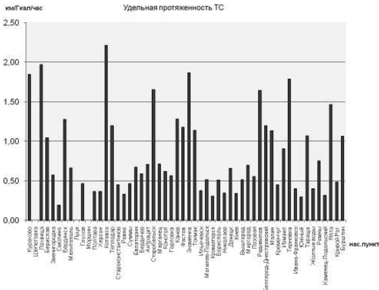
Рис. 4. Удельная протяженность тепловых сетей
