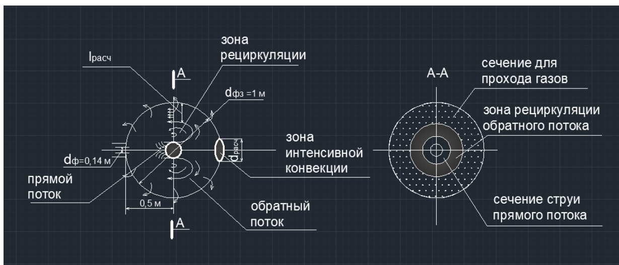
Рис.1 – Зоны теплообмена в фурменной зоне
