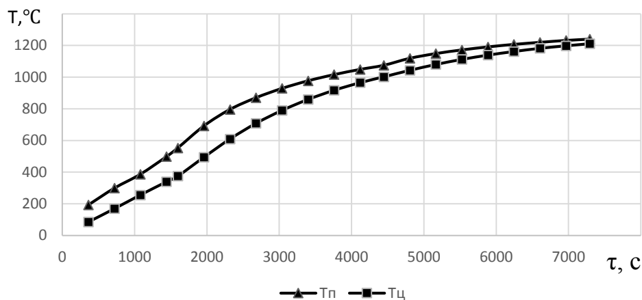
Рис. - Нагрев заготовки толщиной 0,21 \text{ м} .
