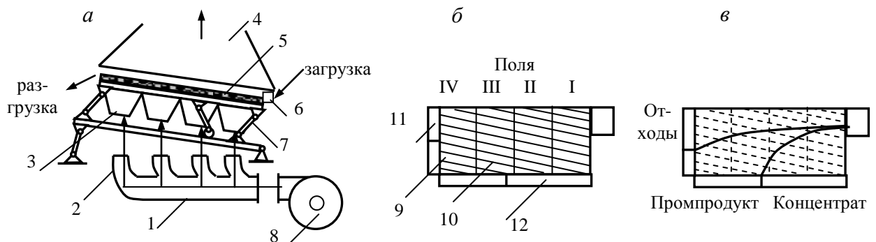
Рисунок 2. Схема вибрационного пневматического сепаратора: а – вид сбоку; б – вид деки сверху, в - зоны выделения продуктов на деке сепаратора
