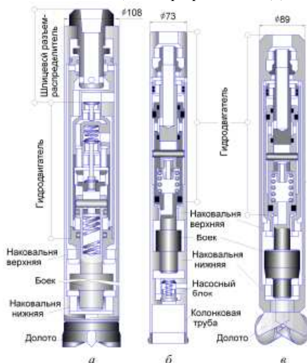
Принципиальные схемы ГДД для бурения сплошным забоем (а), (в) и колонкового бурения с обратной призабойной промывкой (б)
