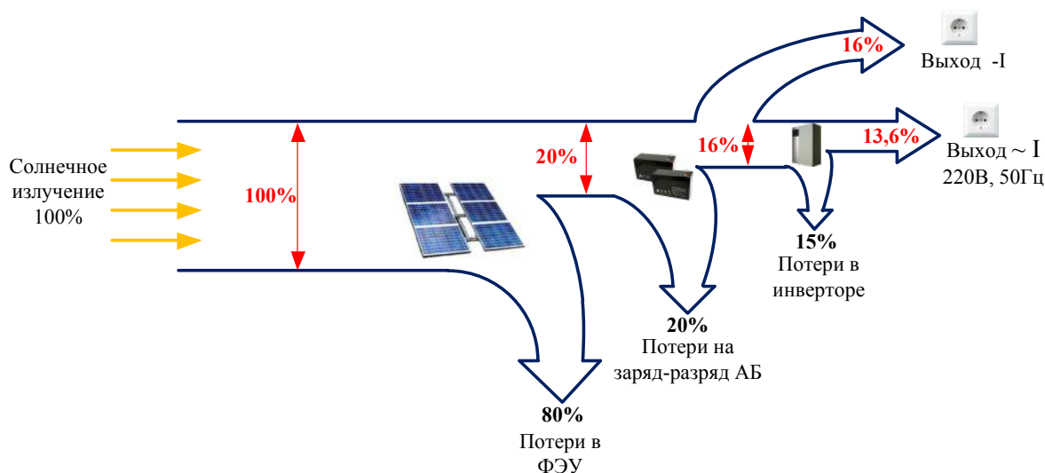
Рис. 2 – Энергетическая диаграмма преобразования солнечного излучения (СИ) в электрическую энергию (ЭЭ)
