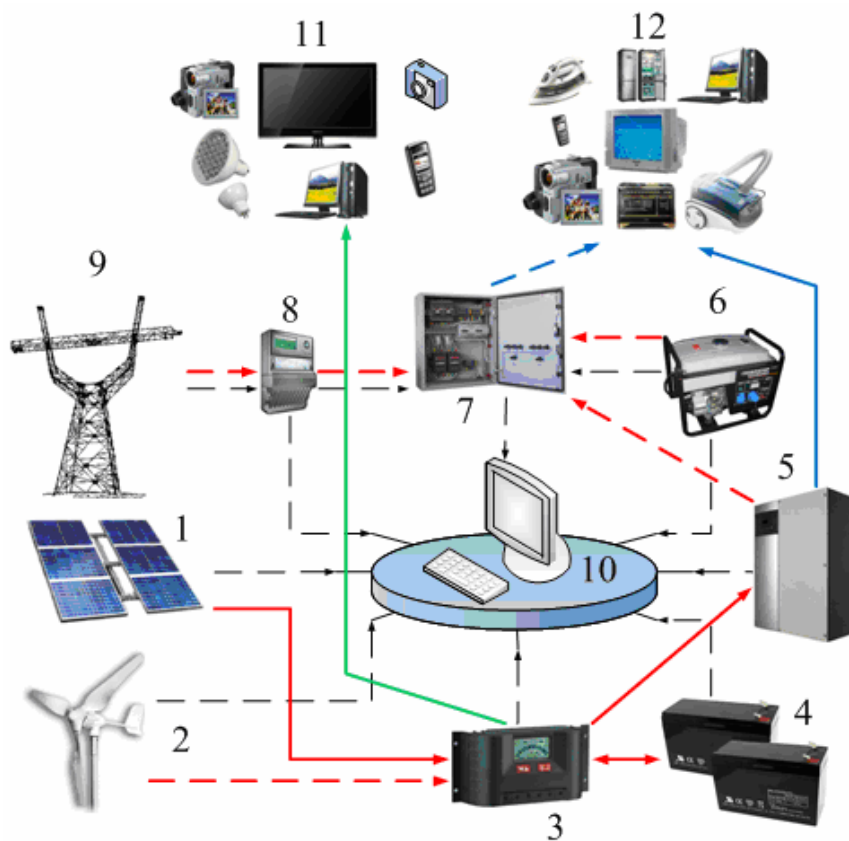
Рис. 1 - Структурная схема системы автономного электроснабжения:
