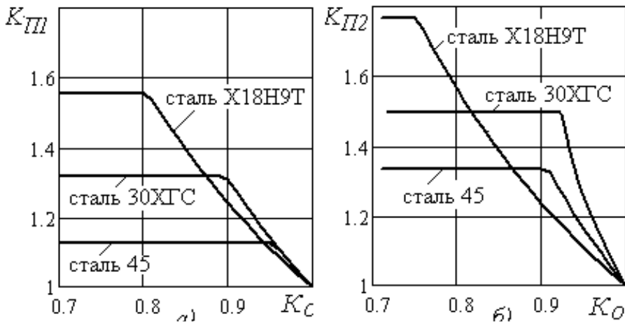
Рис. 2. Графіки зміни коефіцієнтів підвищення продуктивності K_{II} від коефіцієнта зниження температури K_O для різних сталей під час чорнової обробки – а) та чистової обробки – б)
