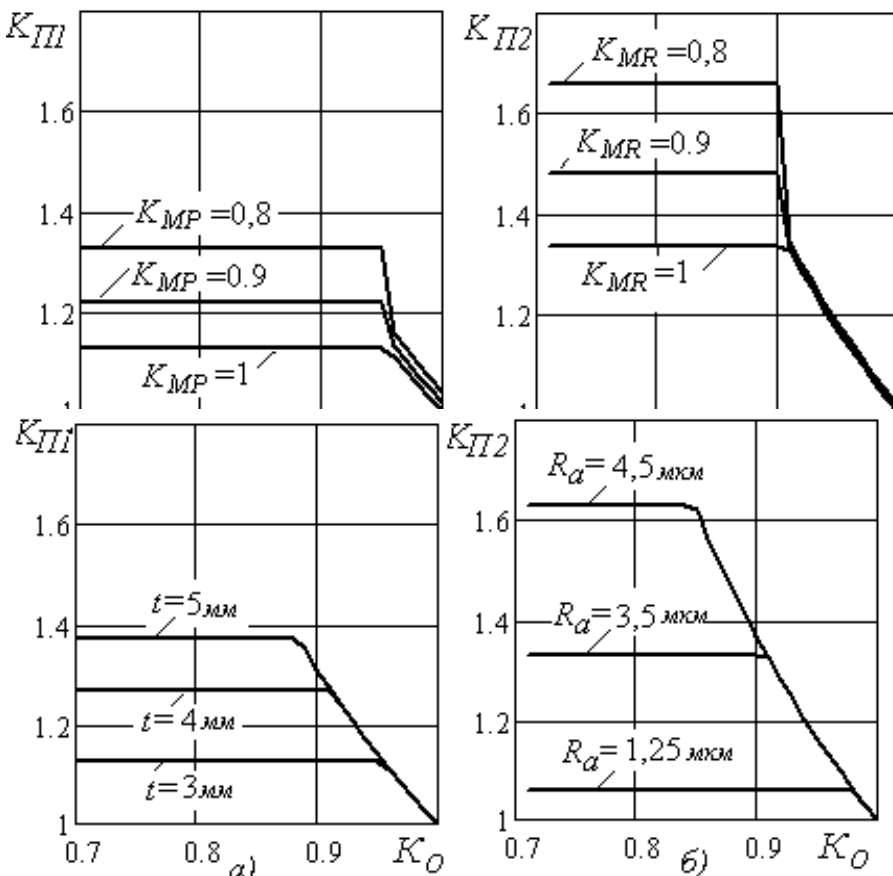
Рис. 4. Графіки зміни коефіцієнтів підвищення продуктивності K_{II} від коефіцієнта зниження температури K_O для різних глибин різання t та шорсткостей поверхні R_a під час чорнової обробки а) та чистової обробки – б)
