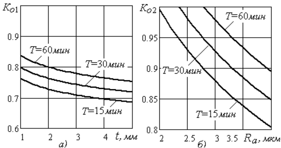
Рис. 1. Графіки зміни граничних коефіцієнтів K_{O1} та K_{O2} від глибини різання t під час чорнкової обробки – а) та шорсткості обробленої поверхні R_a під час чистової обробки – б)
