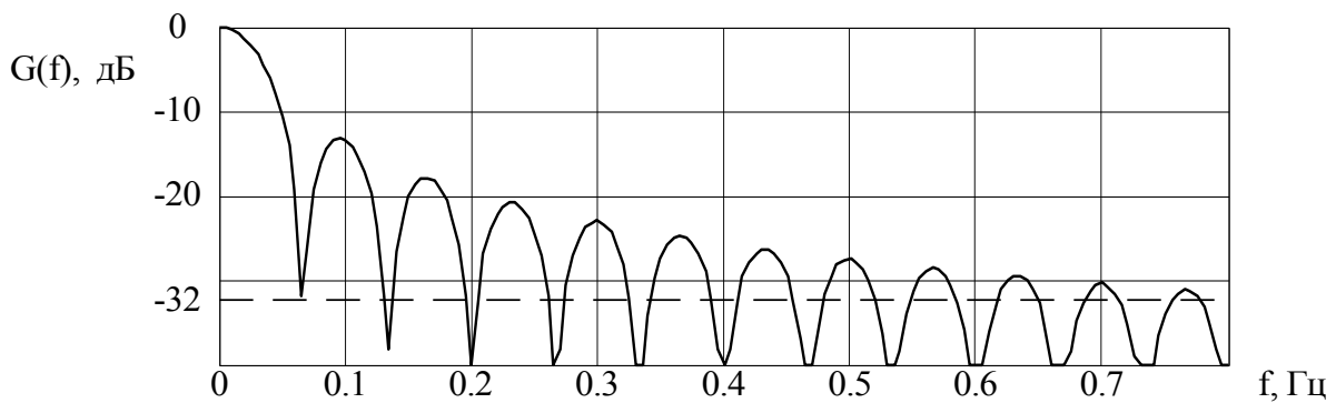
Рисунок 3 – АЧХ при усреднении посредством нахождения среднего арифметического
