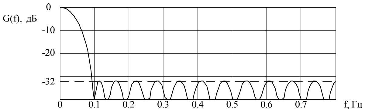
Рисунок 2 – АЧХ временного окна Дольфа-Чебышева.
