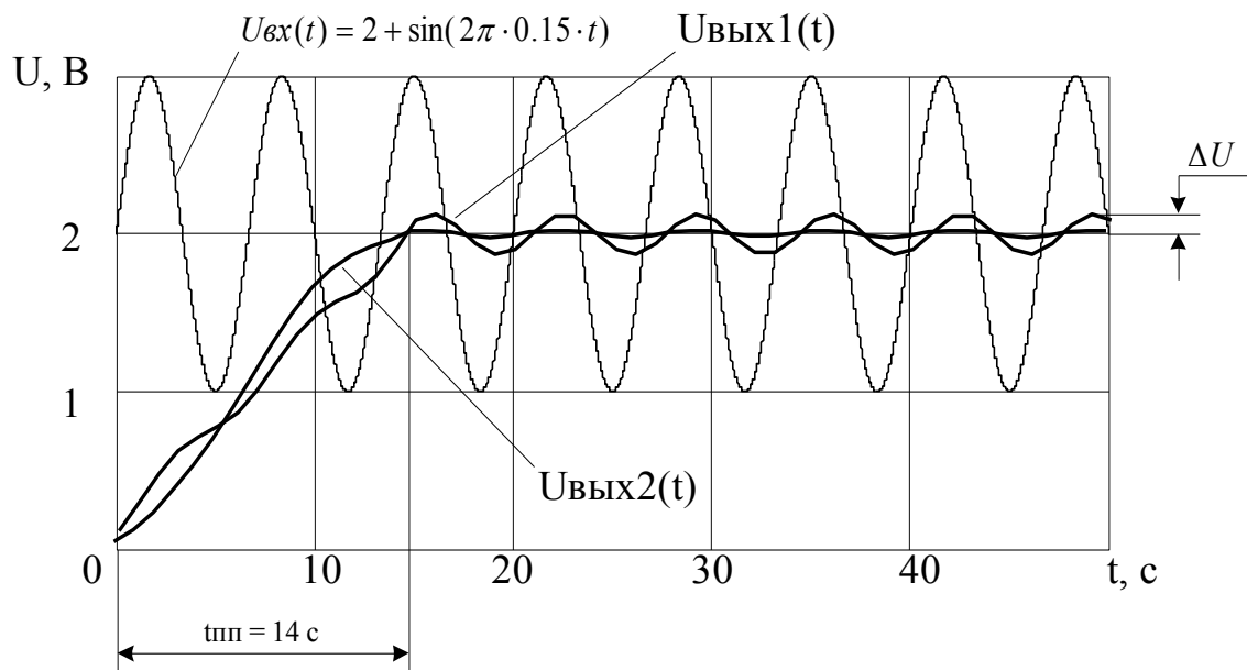
Рисунок 4 – Реакции фильтров на входное воздействие U_{вх}(t) :
