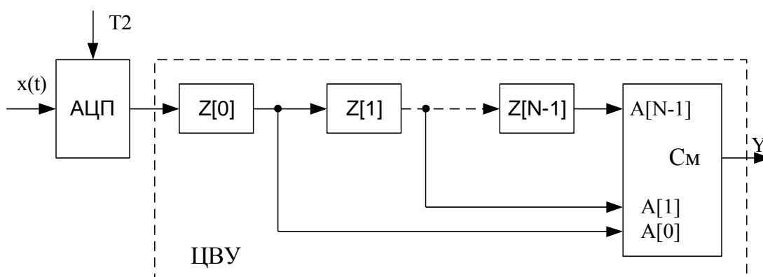
Рисунок 1 – Структурная схема цифрового КИХ-фильтра
