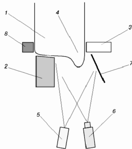
Рис. 3. Система «EVA»: 1 – колесо; 2 – направляющая плита; 3 – защитный рельс; 4 – гребень; 5 – лазер; 6 – камера; 7 – зеркало; 8 – датчик положения колеса
