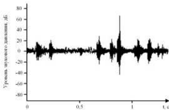
Рис. 6. Звуковая дорожка, записанная при прохождении подвижного состава с дефектом поверхности катания колеса
