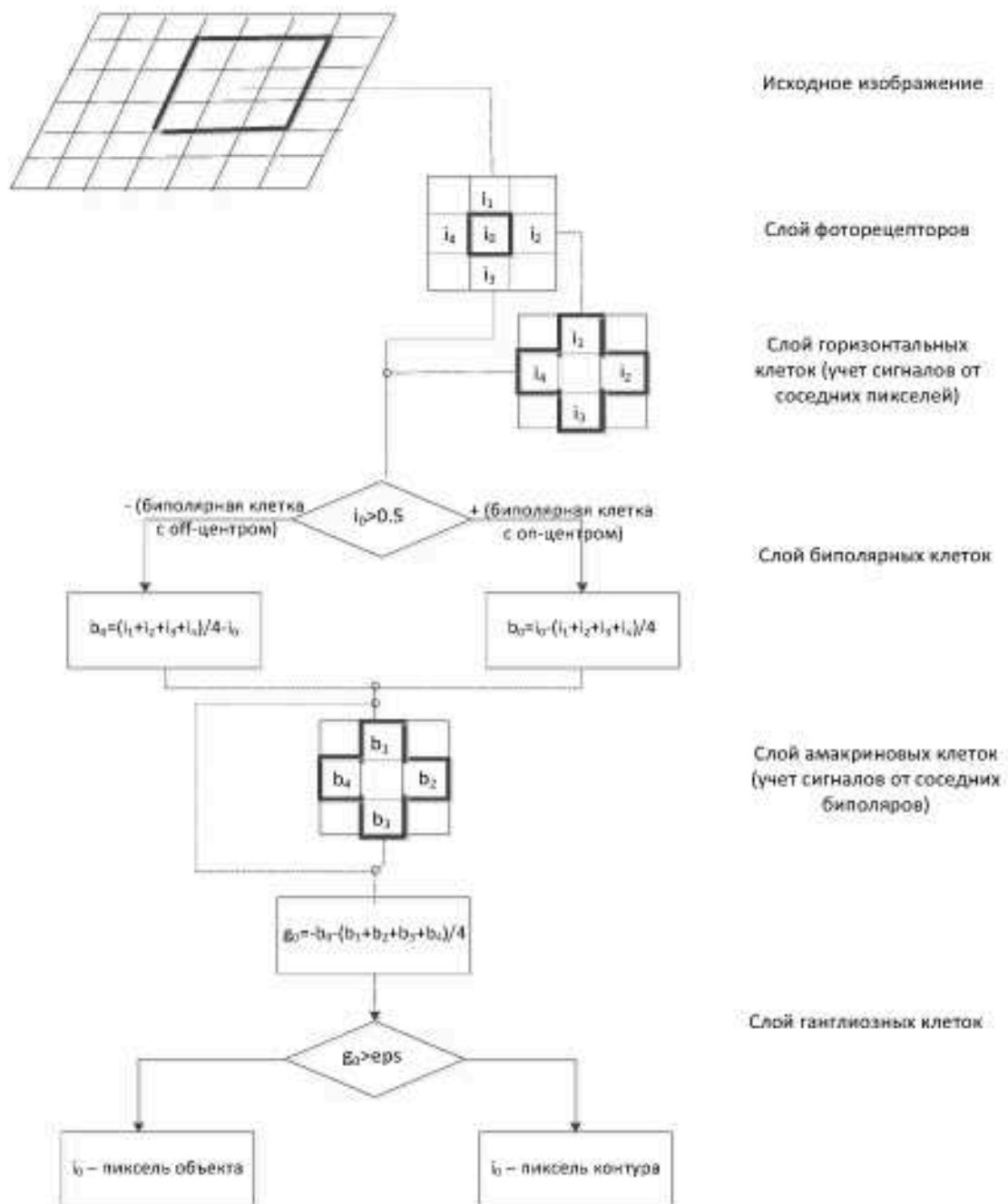
Рисунок 3 – Условная схема метода выделения контуров
