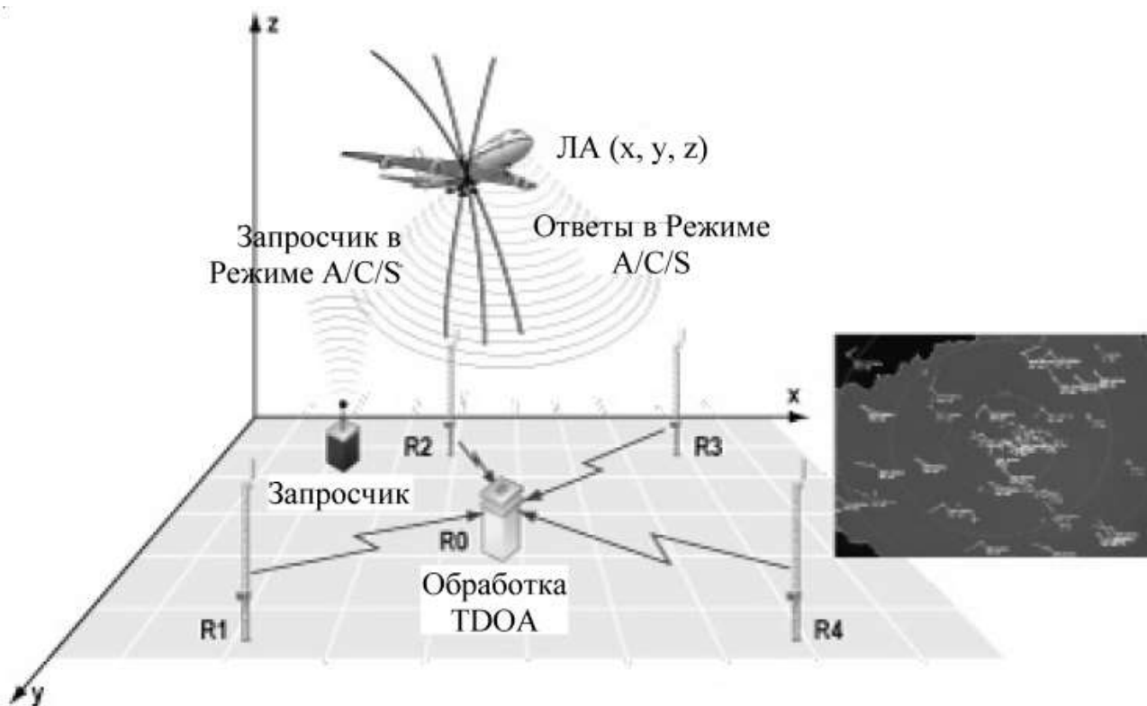
Рис. 1. Принцип действия системы мультilaterации MLAT.
