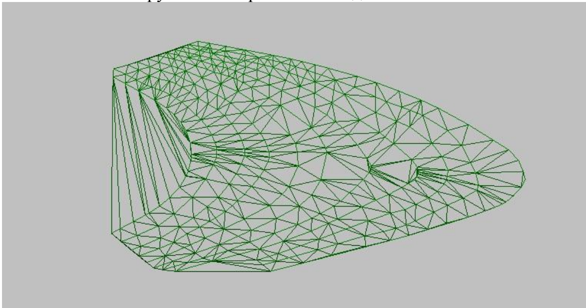
Рис.1 - Каркасная модель поверхности пласта
