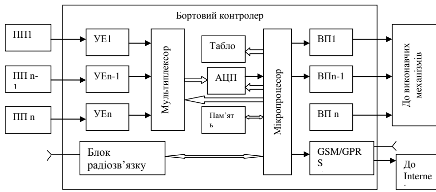
Рис. 1. Структурна схема мобільного обладнання
