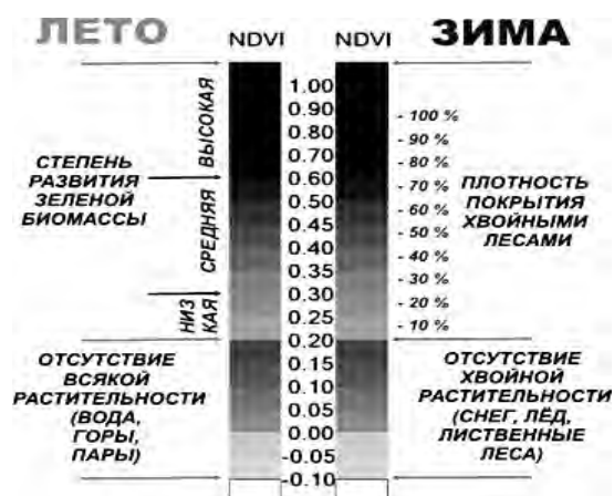
Рис. 10. Значения NDVI и соответствующие им типы растительного покрова
