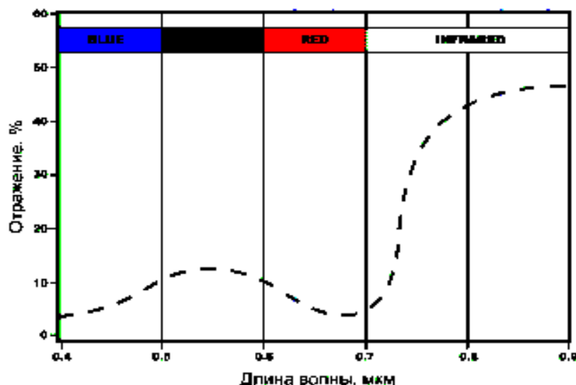
Рис. 1. Участки характеристической кривой отражения растительности (усредненной), используемые для расчета NDVI с помощью данных MODIS
