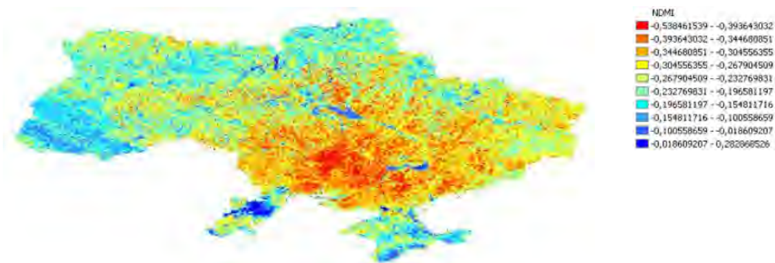
Рис. 6. Карта влагосодержания почвы на территории Украины за 23 мая 2007 г. по данным КА Terra (MODIS)
