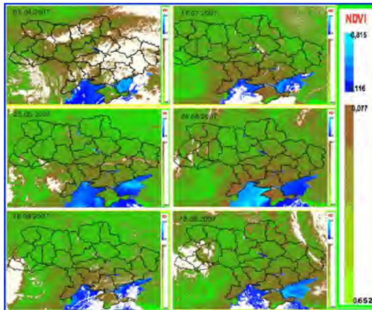
Рис. 3. Индекс вегетации растительности на территории Украины за 2007 год
