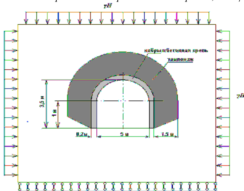
Рис. 2. Расчетная схема выработки с набрызгбетонной крепью, толщиной 20 см и тампонажем закрепного пространства на глубину 1,5 м
