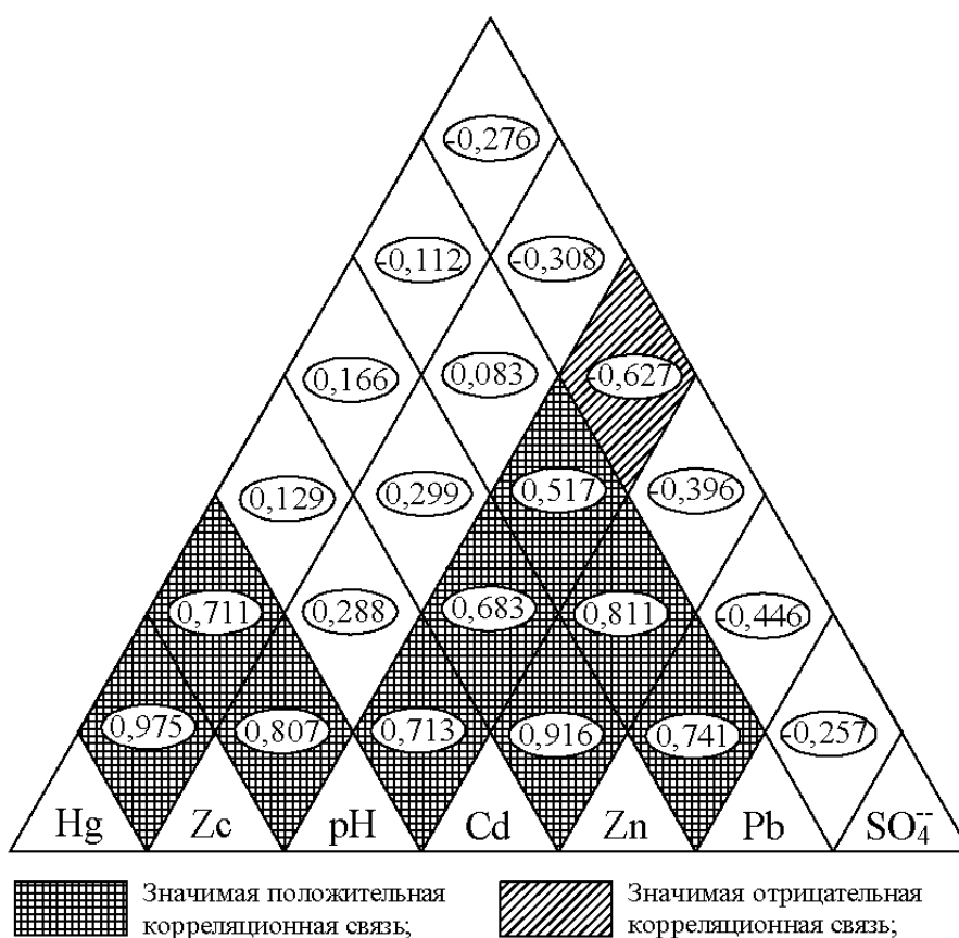
Рис. 3. Диаграмма корреляционных связей между основными показателями загрязнения почв пробы №1 ( R_{\alpha=0,05} \geq 0,513 , n=13 )
