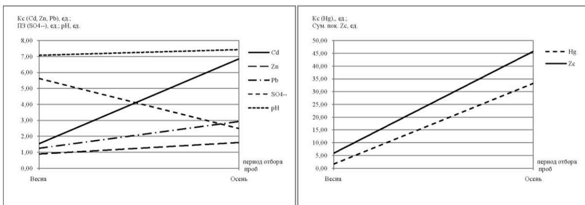
Рис. 2. Диаграмма средних значений основных показателей загрязнения почв пробы №1 в весенний и осенний этапы регулярного мониторинга.
