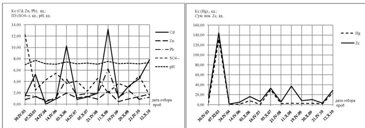
Рис. 1. Временная динамика основных показателей загрязнения почв в пробе №1 регулярного мониторинга.
