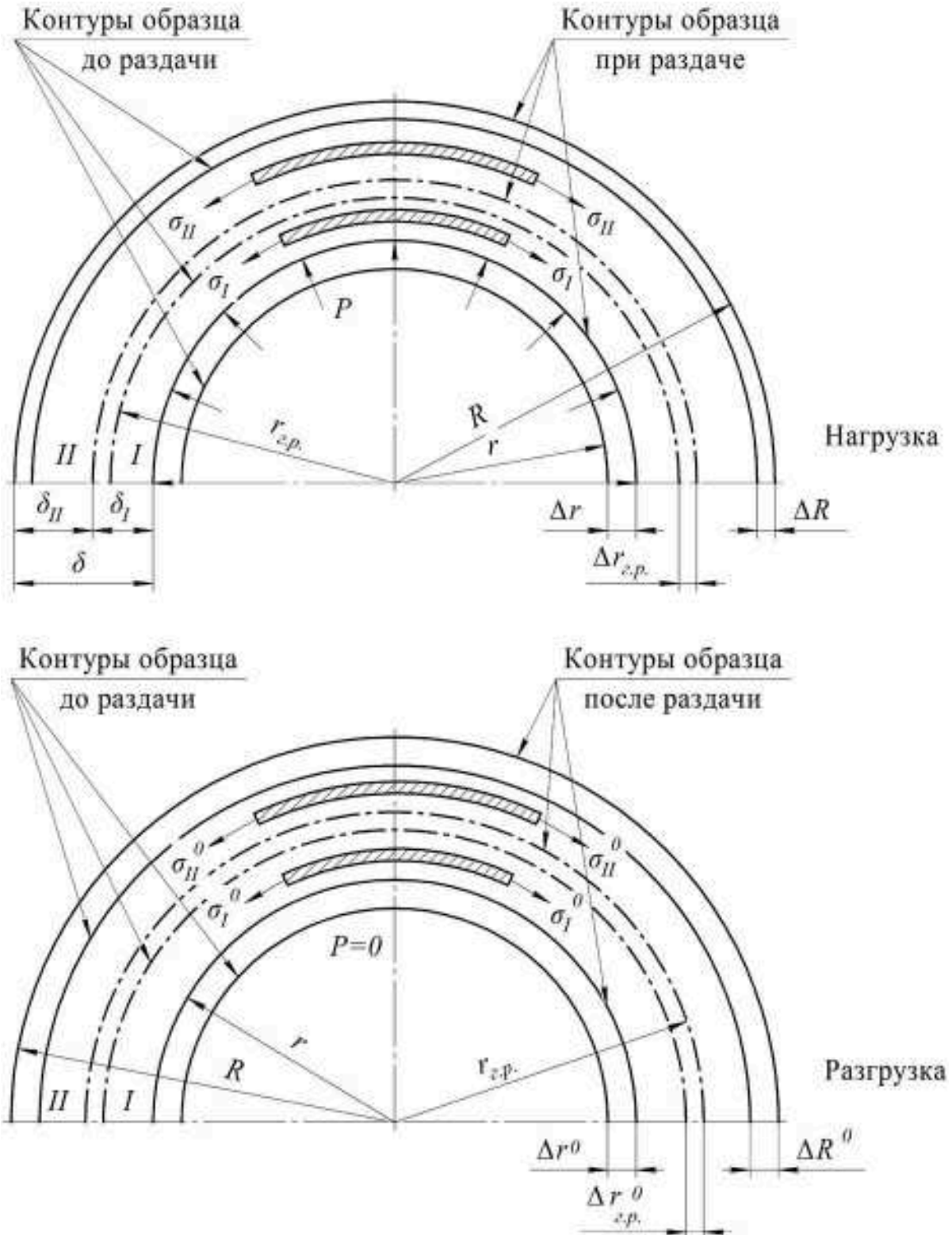
Рисунок 1 – Схема напряжённого состояния образцов
