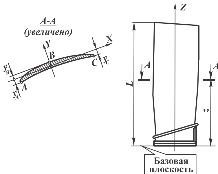
Рис. 1. Лопатка 3-й ступени компрессора ГТД ТВЗ-117
