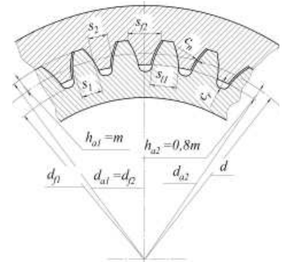
Рисунок 4 – Тангенциальная модификация зубьев
