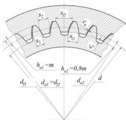
Рисунок 1 – Традиционные параметры зубчатого венца
