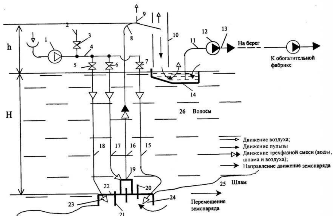
Рисунок 2 – Гидравлическая схема ЭЗК
