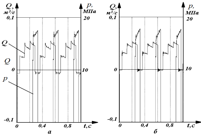
Рис. 3 – Изменения давления p перед насадком и расхода Q на выходе из аккумулятора для гидроимпульсатора: a – традиционной схемы; б – со струйным диодом на ударном трубопроводе.
