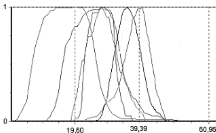
Рисунок 1 – Терм-множество лингвистической переменной «Суммарная ароматика»
