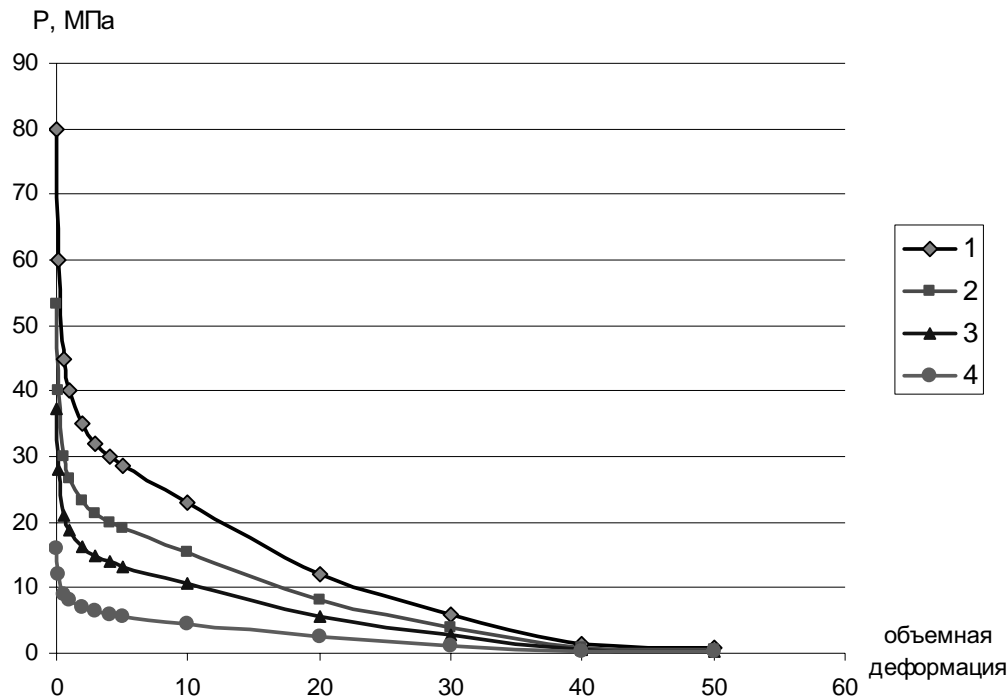
Рис. 2 – Залежність тиску, розвиваемого НРС в залежності від процентного складу SiO_2 при обмеженні можливості об'ємної деформації до 5; 10; 20 і 30% (соответственно кривые 1, 2, 3 и 4).
