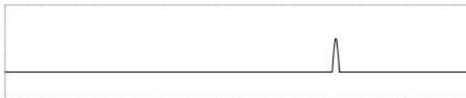
Рис. 22. Изолированная функция
