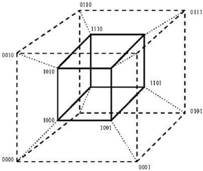
Рис. 19. Четырехмерный куб
