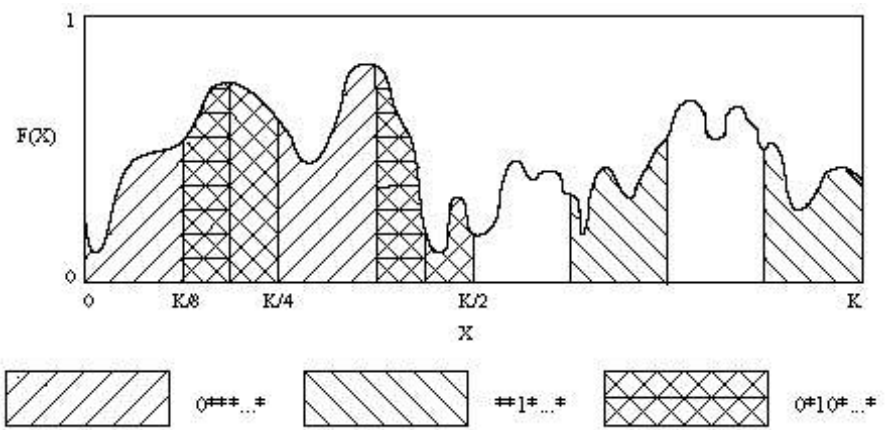
Рис. 20. Разбиение пространства
