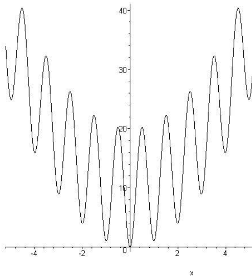
Рис. 21. Функция Растригина
